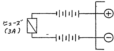
接続図
