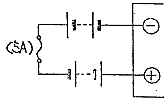
接続図
