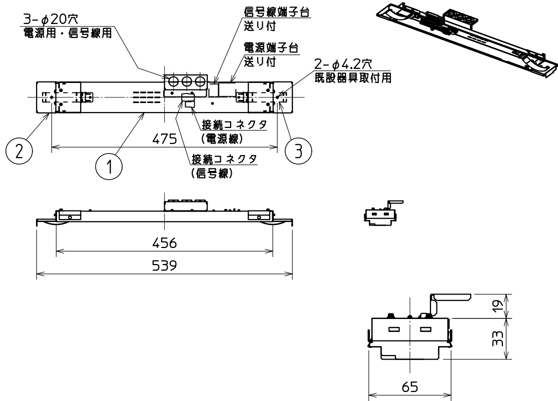
側面詳細図
