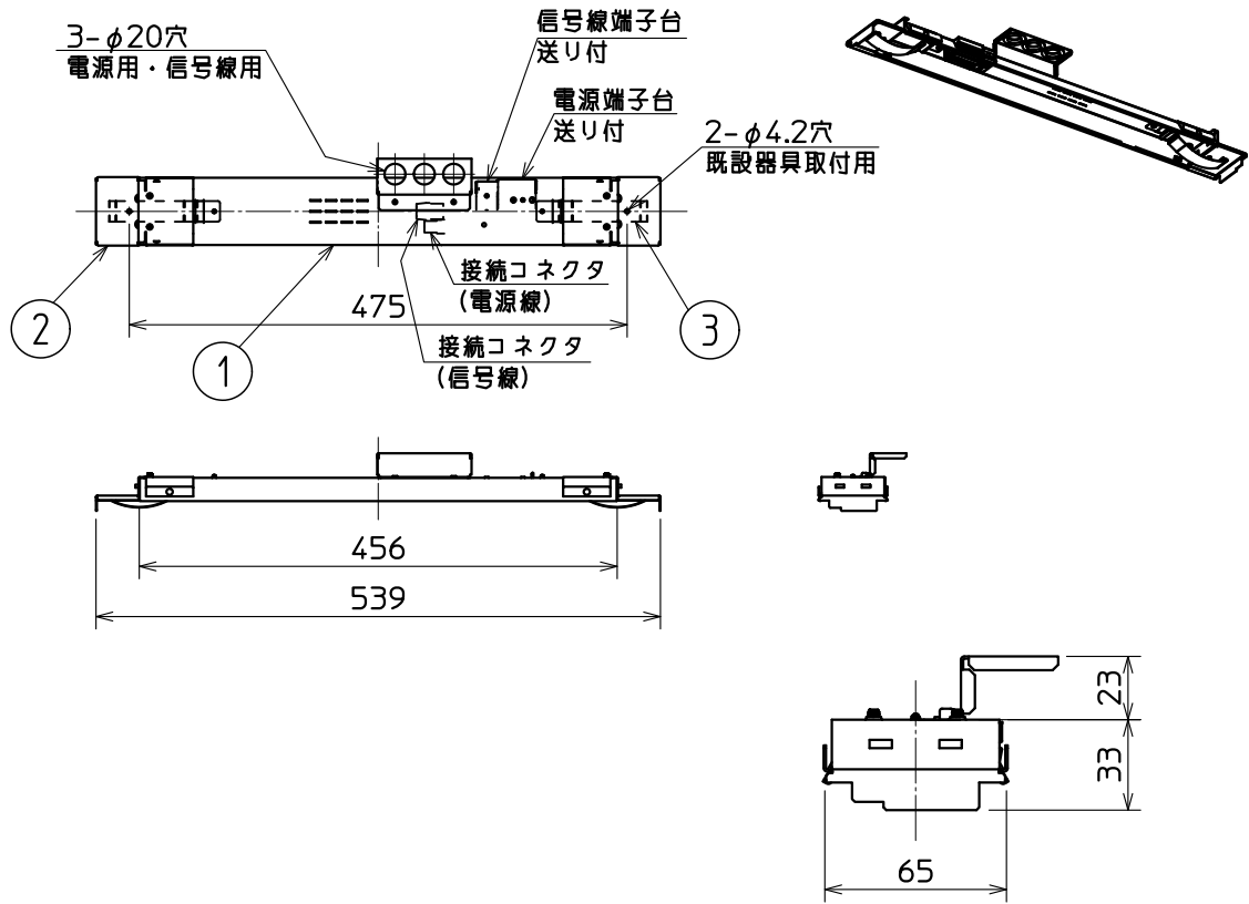
側面詳細図
