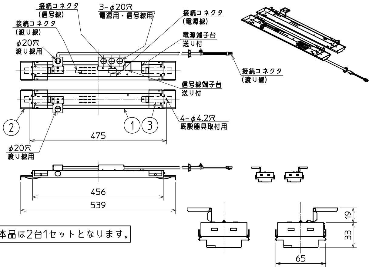
側面詳細図
