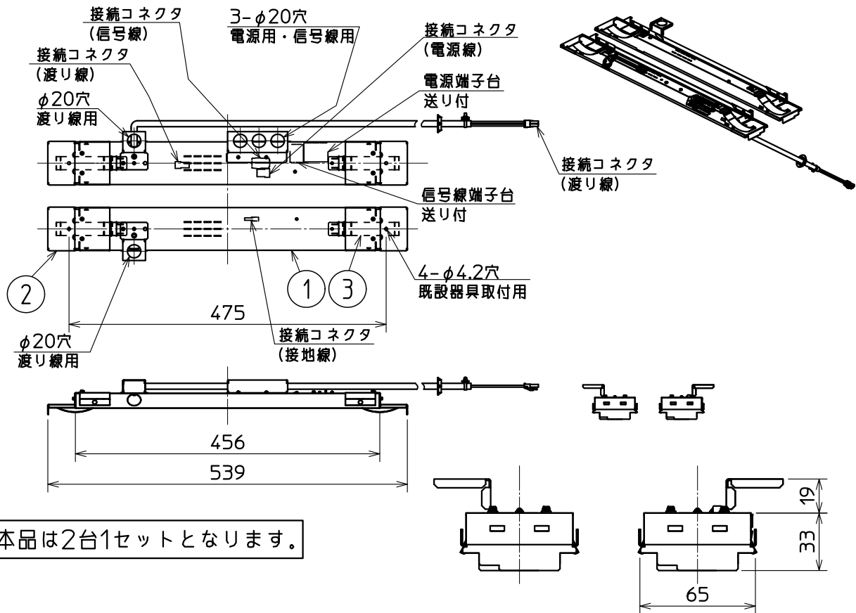
側面詳細図
