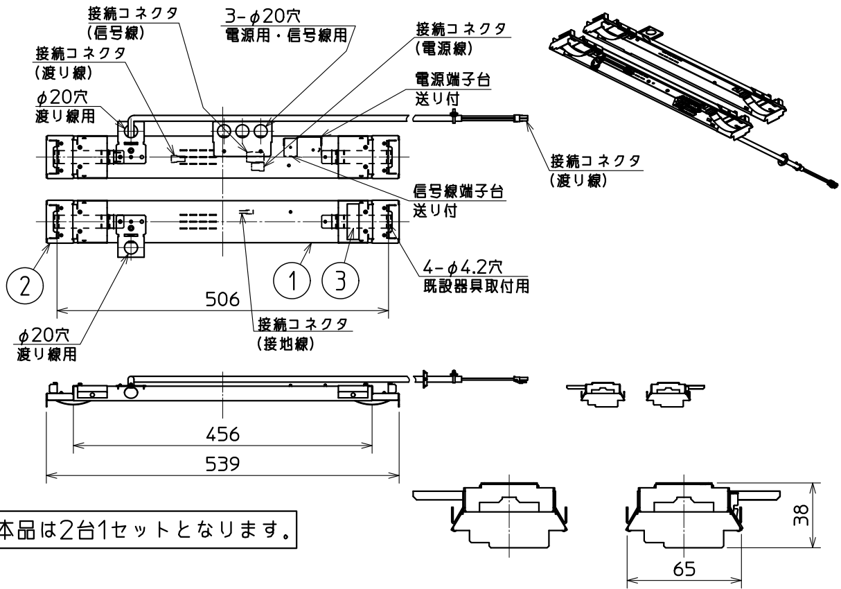
側面詳細図
