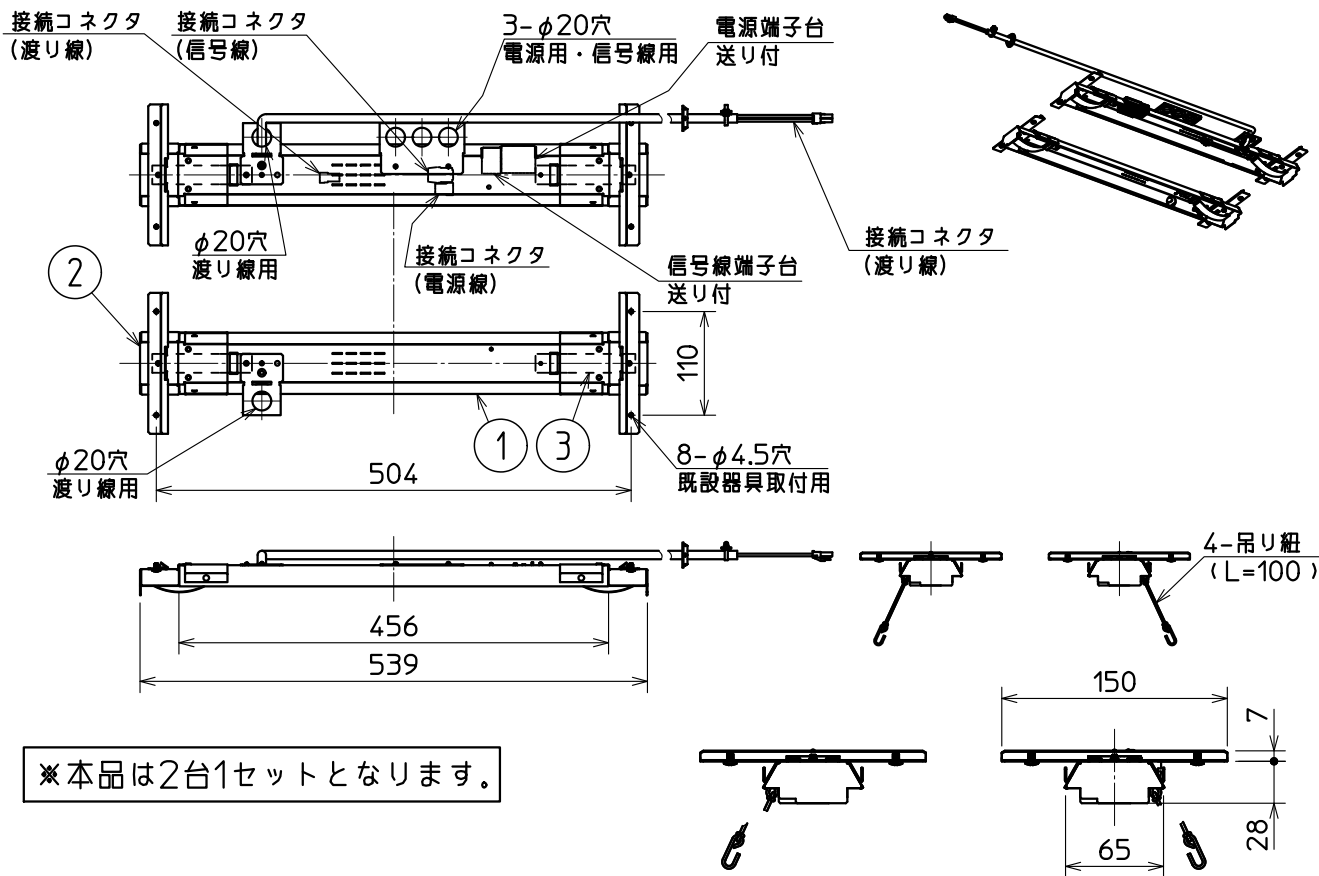
側面詳細図
