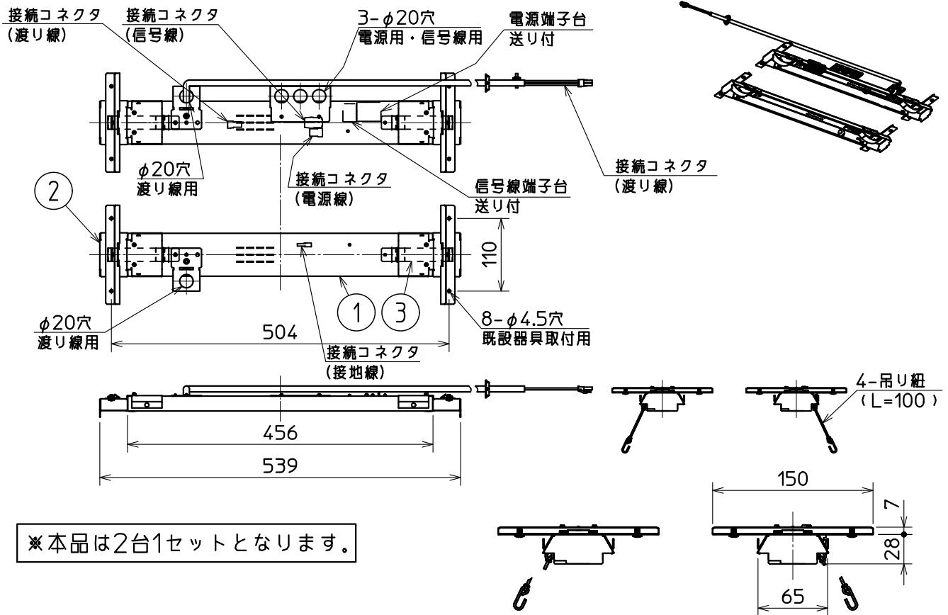
側面詳細図
