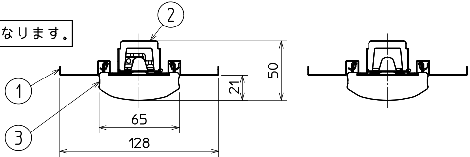
側面詳細図
