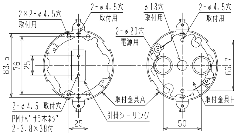
取付寸法図(1)
