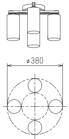
灯具外径寸法
