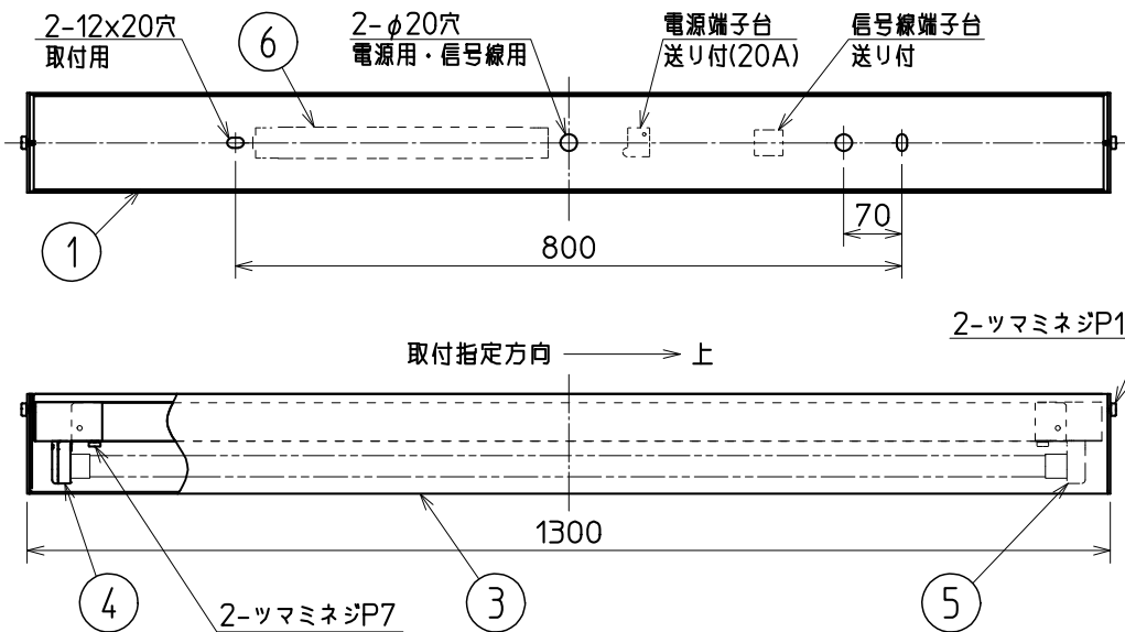
断面詳細図
