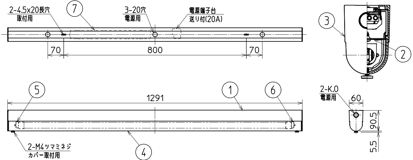
断面詳細図
