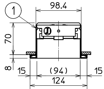
側面詳細図
