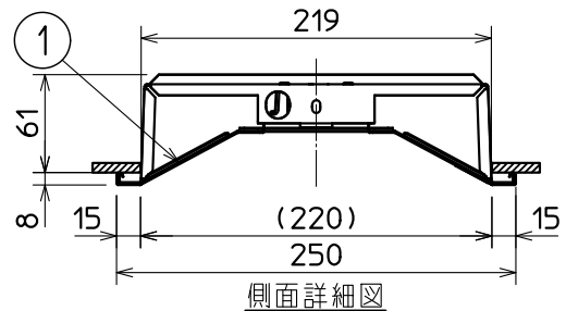
側面詳細図
