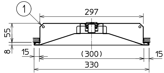
断面詳細図
