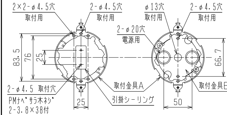
取付寸法図(1)
