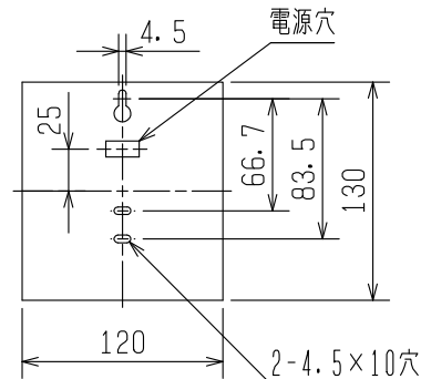
取付寸法図
