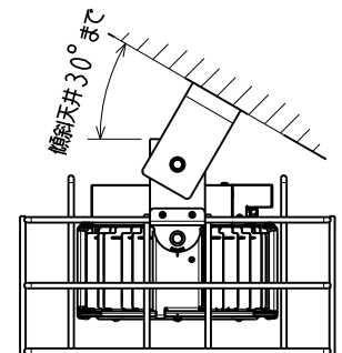
取付要領図
