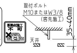
器具取付ボルト長さ
