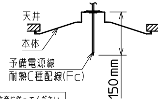
予備電源線器具内引込長さ(推奨)
