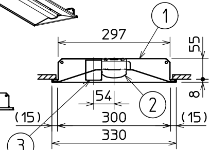
断面詳細図
