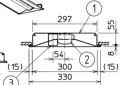
断面詳細図
