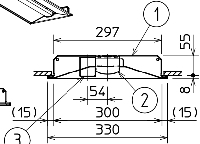
断面詳細図
