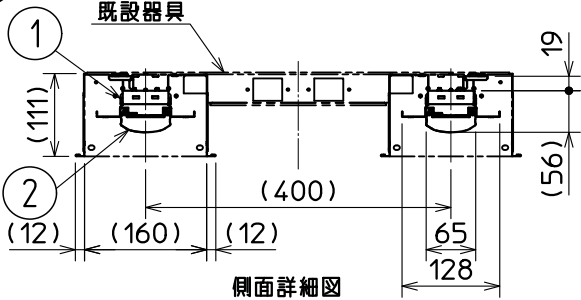
側面詳細図
