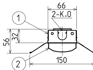
側面詳細図
