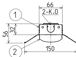
側面詳細図
