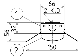
側面詳細図
