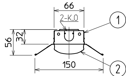
側面詳細図
