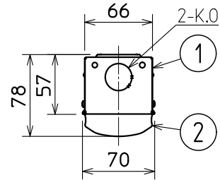
側面詳細図
