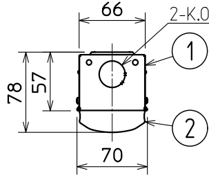
側面詳細図
