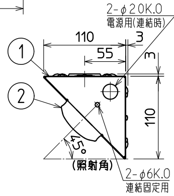
側面詳細図
