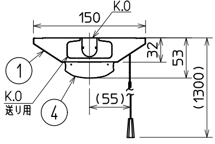
側面詳細図
