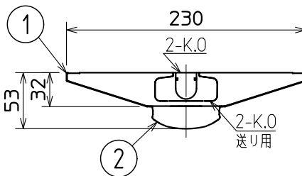
側面詳細図
