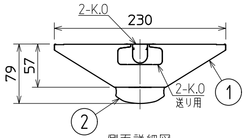
側面詳細図
