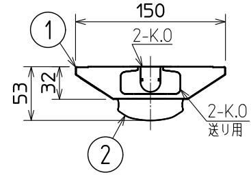
側面詳細図
