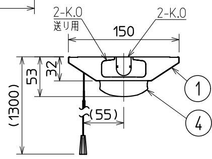
側面詳細図
