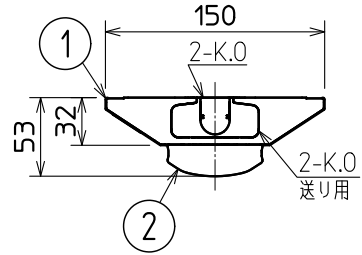
側面詳細図
