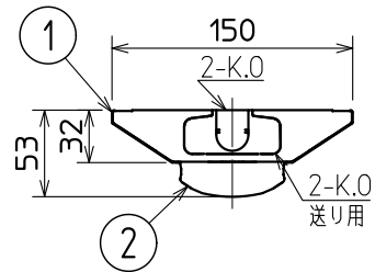
側面詳細図
