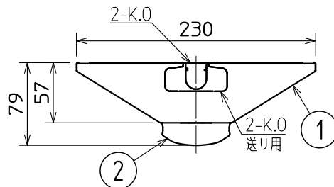
側面詳細図
