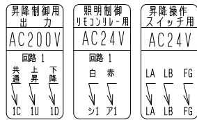
端子配列図
