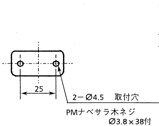
引掛シーリング取付寸法図
