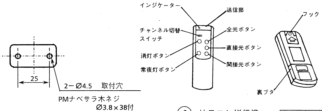
引掛シーリング取付寸法図
