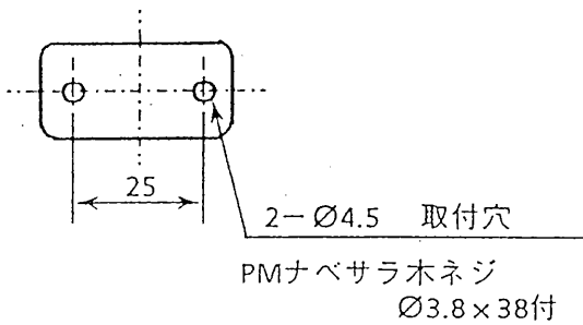
引掛シーリング取付寸法図
