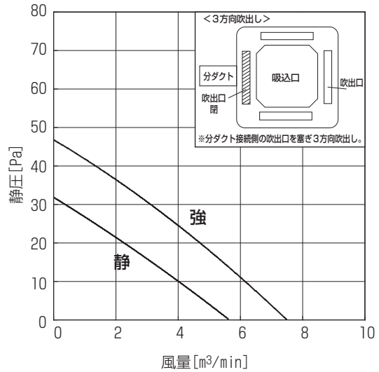
●3方向吹出し(ベーン水平)角形ダクト 1方向分岐
