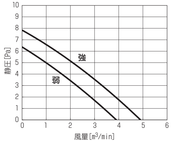
MPS-RP50,56(S)GA(H)2
