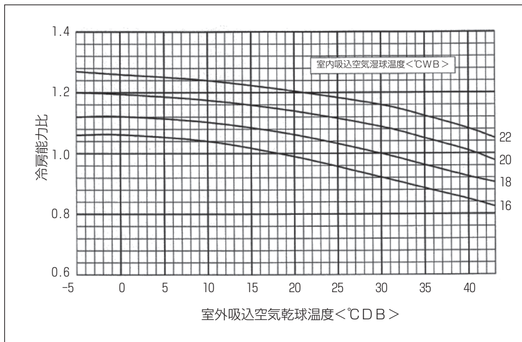
■冷房能力線図 MPUZ-ERP・HA7 / KA, MPU(Z)-RP・HA7
