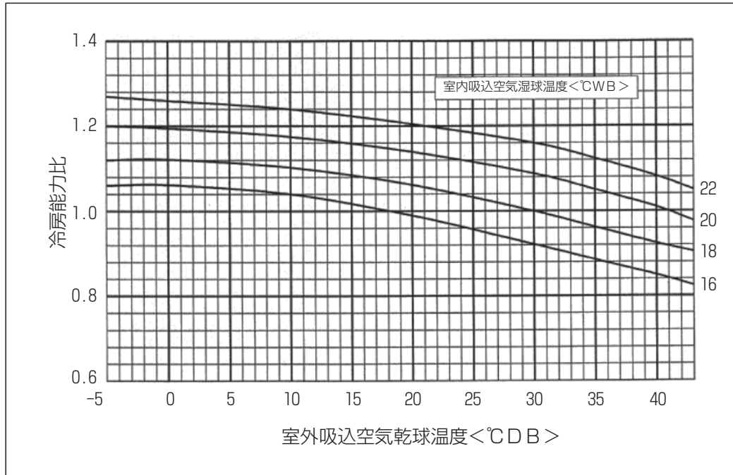
■冷房能力線図 MPUZ-HRP・HA6
