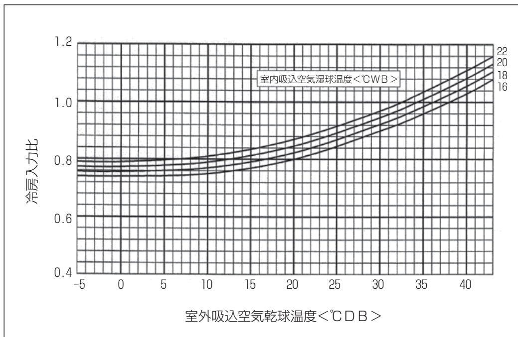
■冷房入力線図 MPUZ-HRP・HA6
