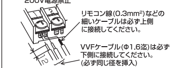
<図1>TB5:端子盤(リモコン伝送線)への配線接続時の注意
