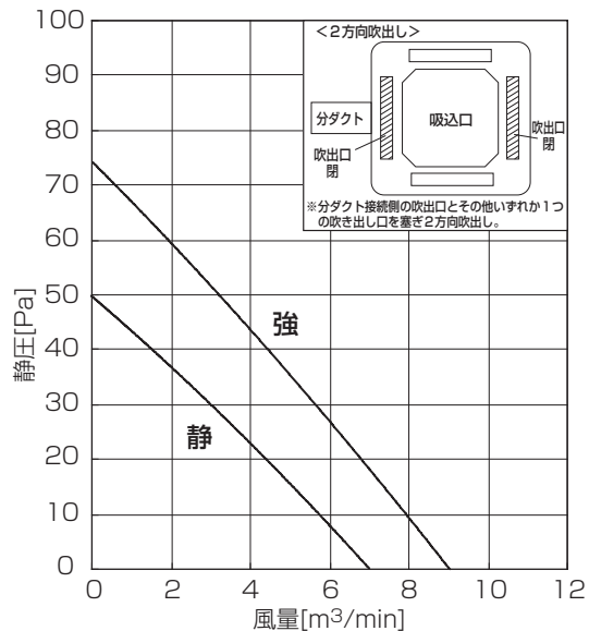
●2方向吹出し(ペーン水平)角形ダクト 1方向分岐
