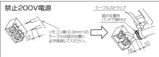
〈図1〉TB5:端子盤(リモコン伝送線)への配線接続時の注意
