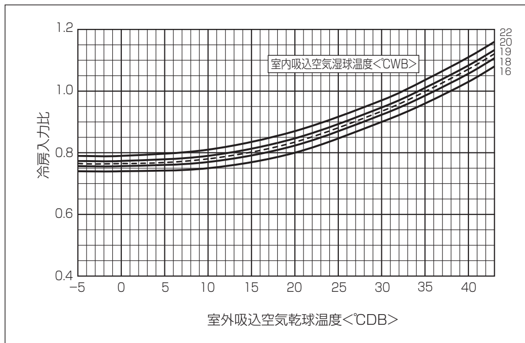
■冷房入力線図 PUZ-HRP・HA12
