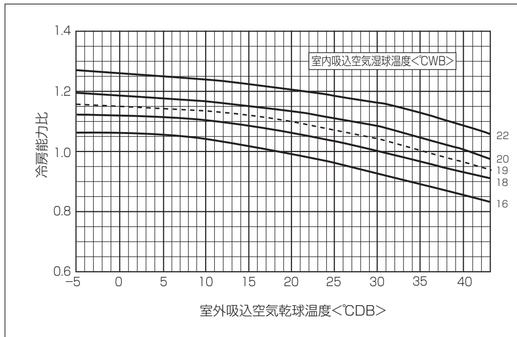
■冷房能力線図 PUZ-HRP・HA12
