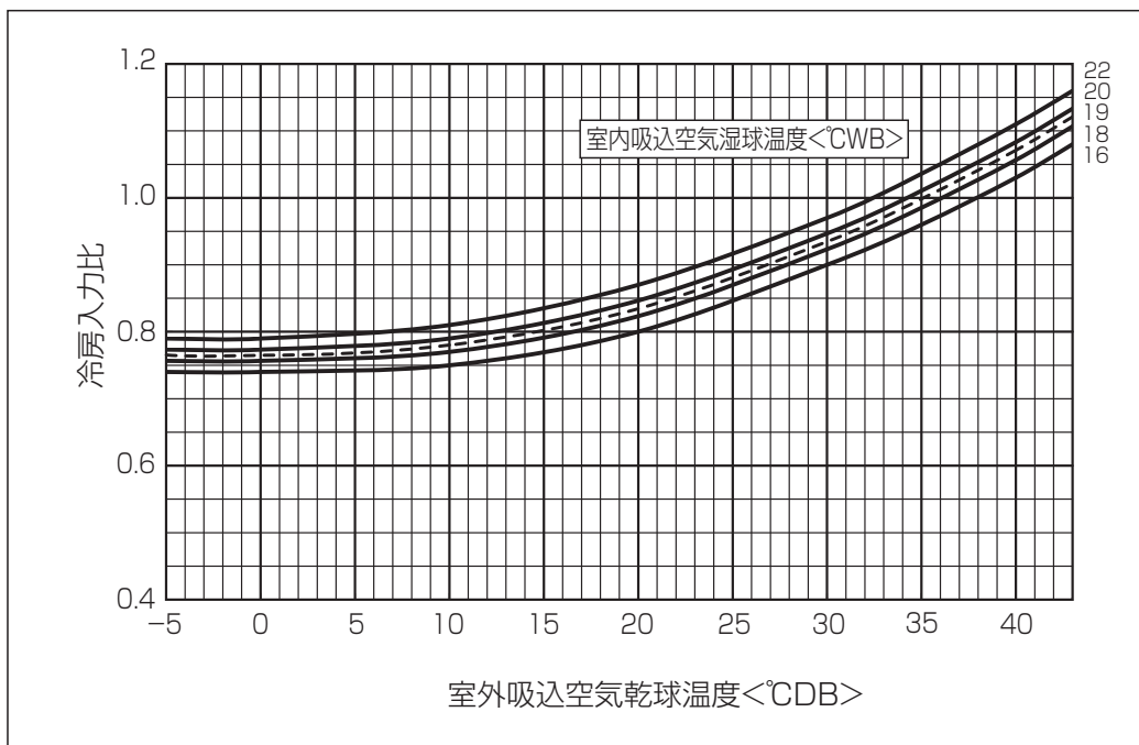
■冷房入力線図 PUZ-HRP・HA9
