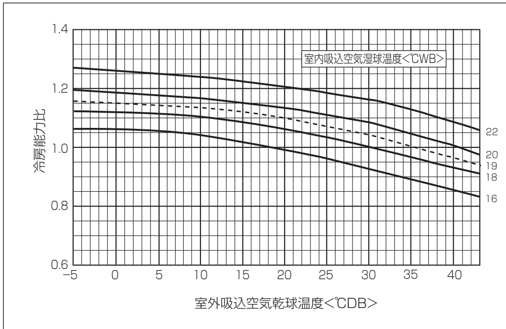
■冷房能力線図 PUZ-HRP・HA9
